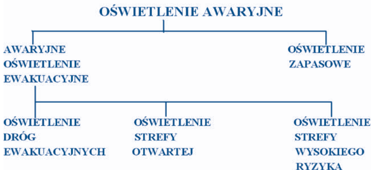
Rys. 1. Rodzaje oświetlenia awaryjnego (wg PN-EN [2])
