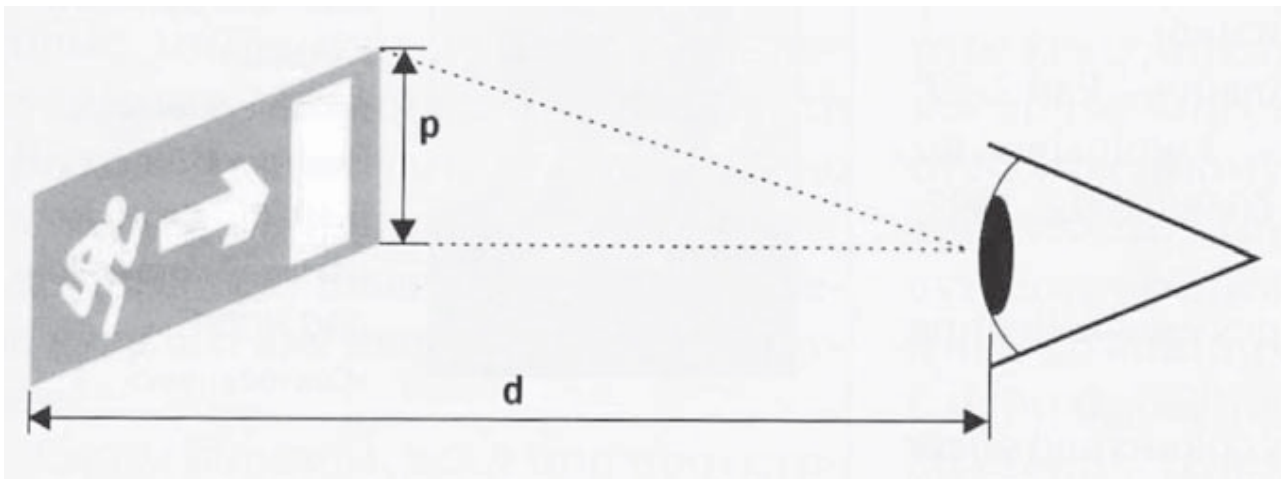
Rys. 5. Odległość widzenia znaków podświetlanych wewnątrz
