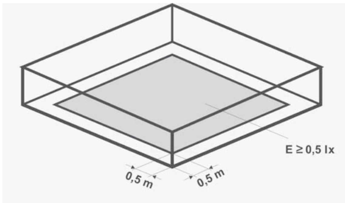
Rys. 4. Znormalizowany obszar dużego pomieszczenia
